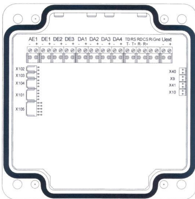
Рис. 2 Расположение разъёмов на плате корректора ЕК260
