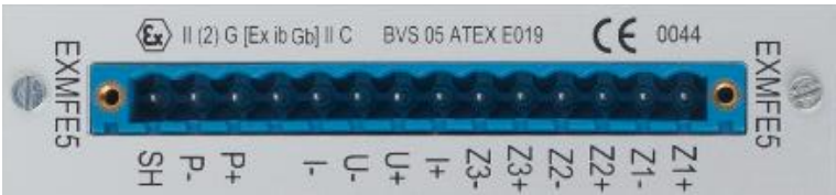
Рисунок 3 Разъем подключения контактов платы входов ExMFE5
