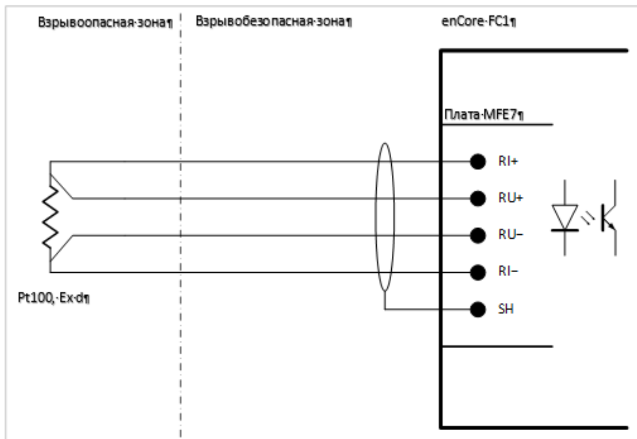
Рисунок 18 Схема подключения преобразователя температуры с HСХ Pt100 к плате MFE7.
