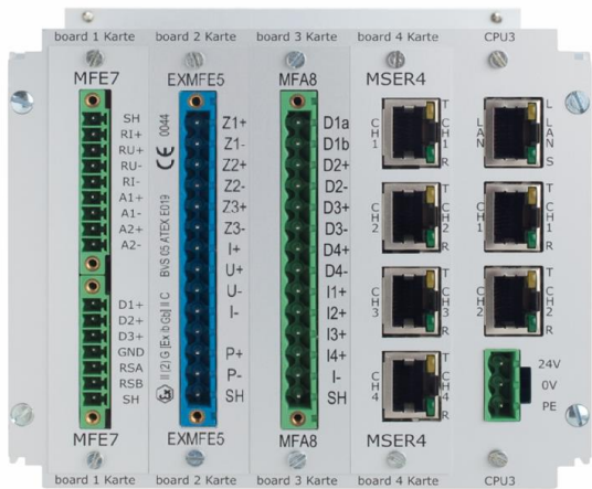
Рисунок 1 Вычислитель enCore FC1, исполнение 1, вид сзади.
