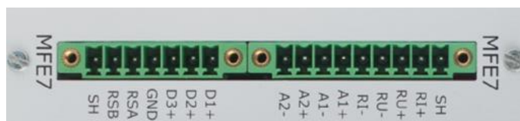
Рисунок 4 Разъемы подключения контактов платы входов MFE7
