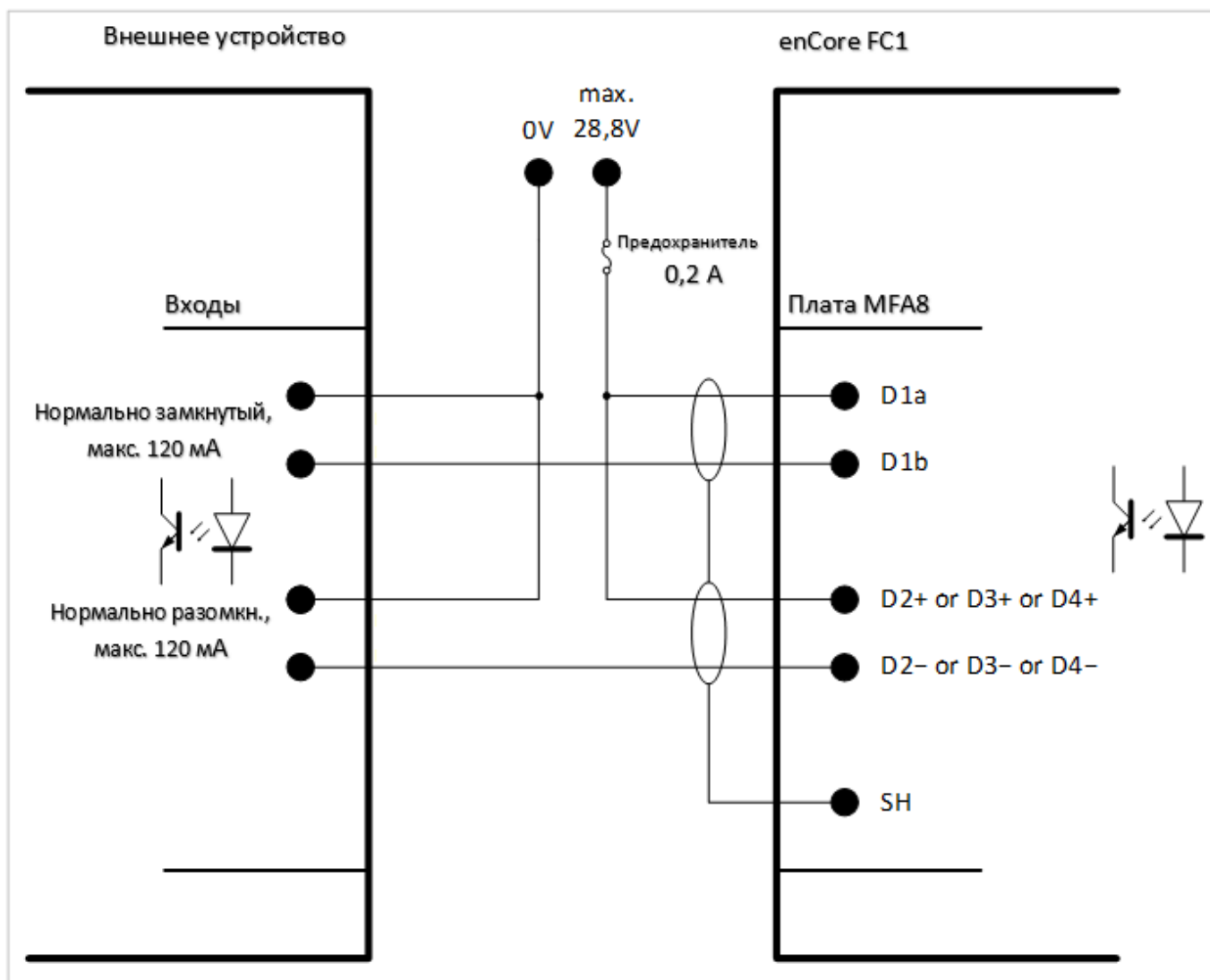
Рисунок 38 Выходы концевой типа платы MFA8
