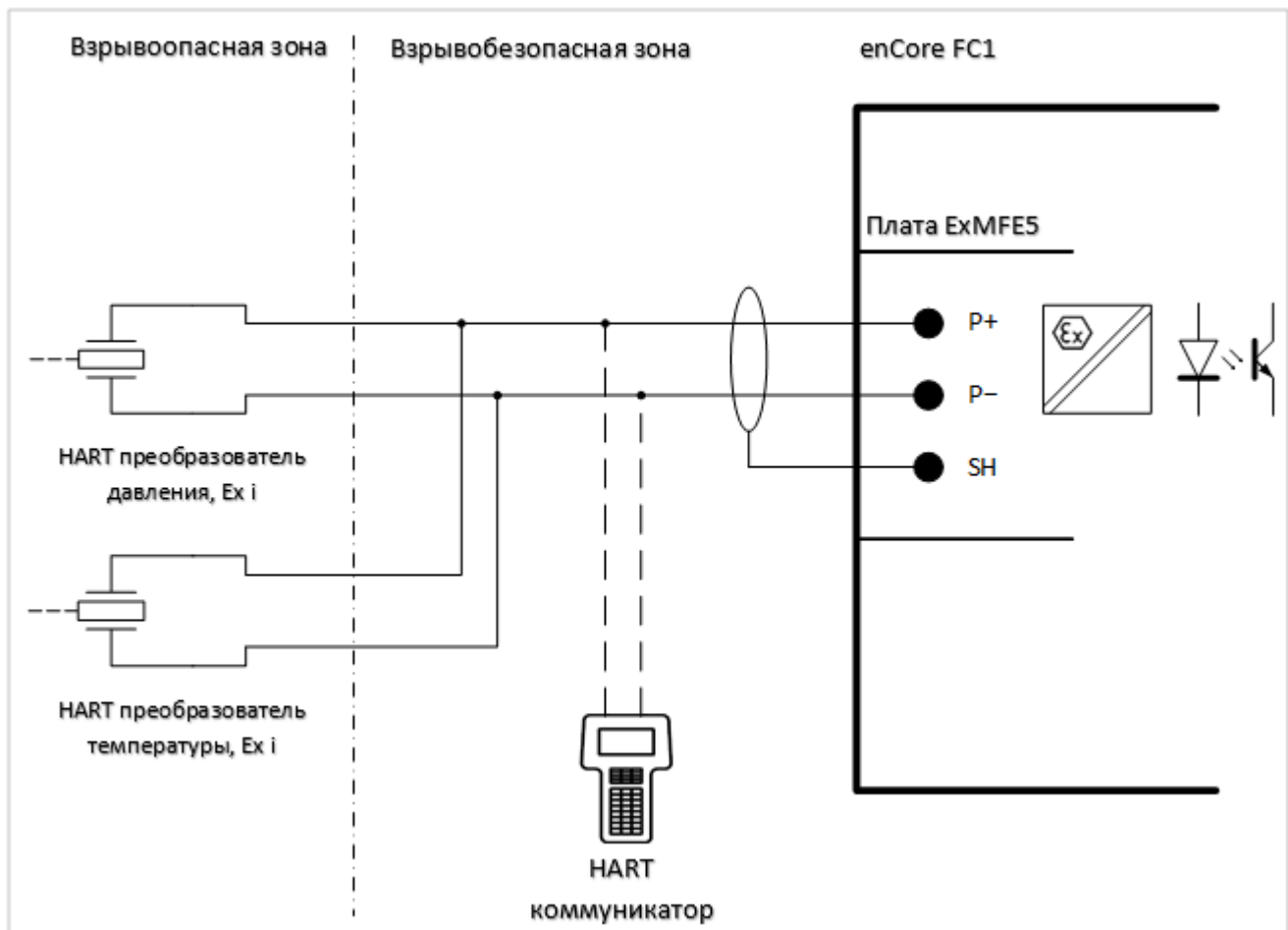
Рисунок 23 Схема подключения преобразователей давления и температуры (Ex i) по протоколу HART к плате ExMFE5.
