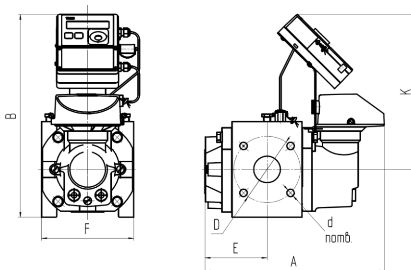
Рисунок 1 Направление потока газа – слева - направо
