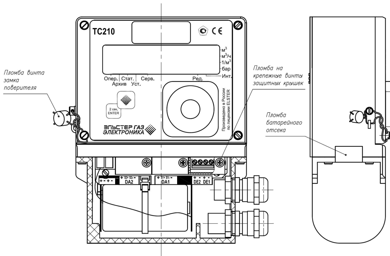
Рис 10. Расположение пломб
