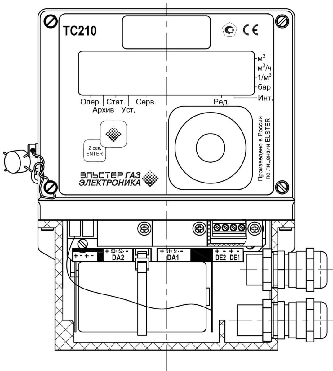
Рис 8. Расположение выводов
