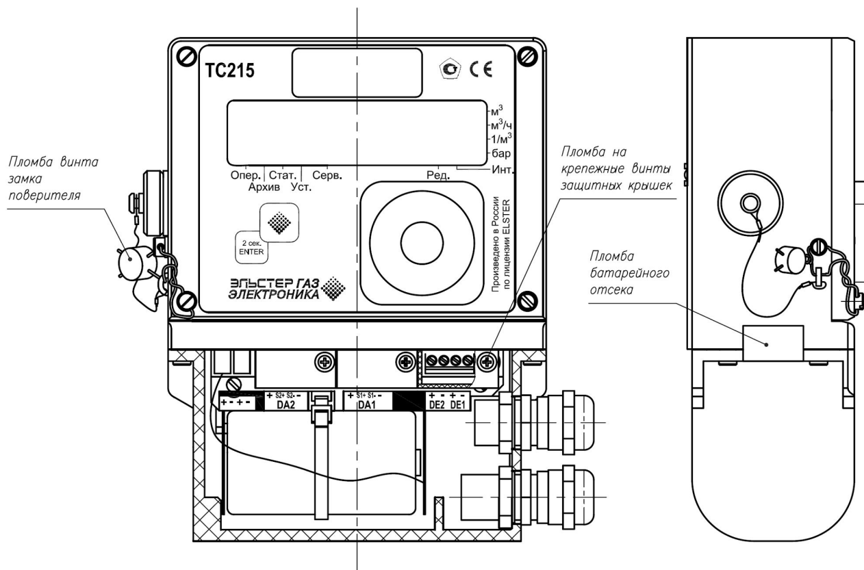
Рис 11. Расположение пломб
