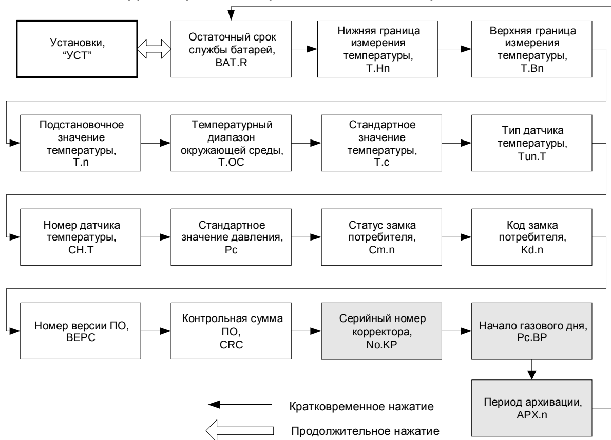
Рис. 6. Меню «Установки»
