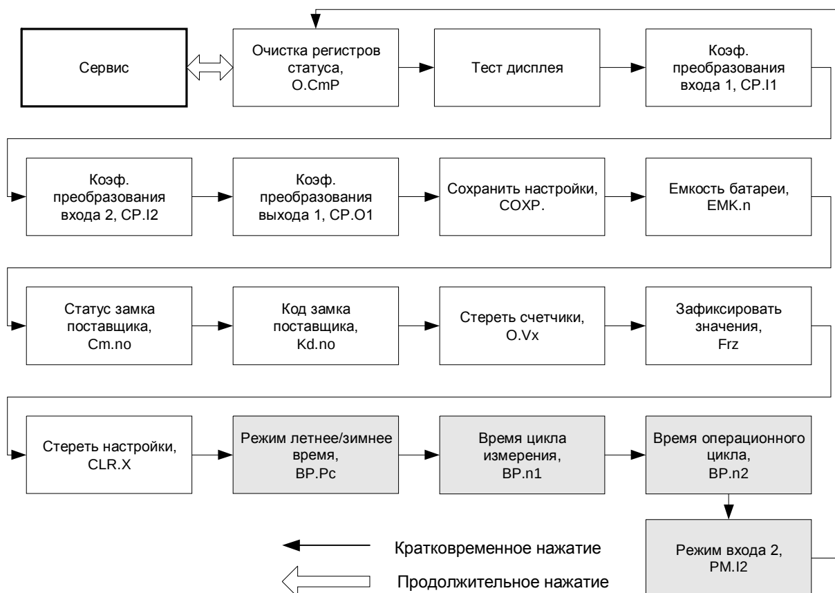
Рис. 7. Меню «Сервис»
