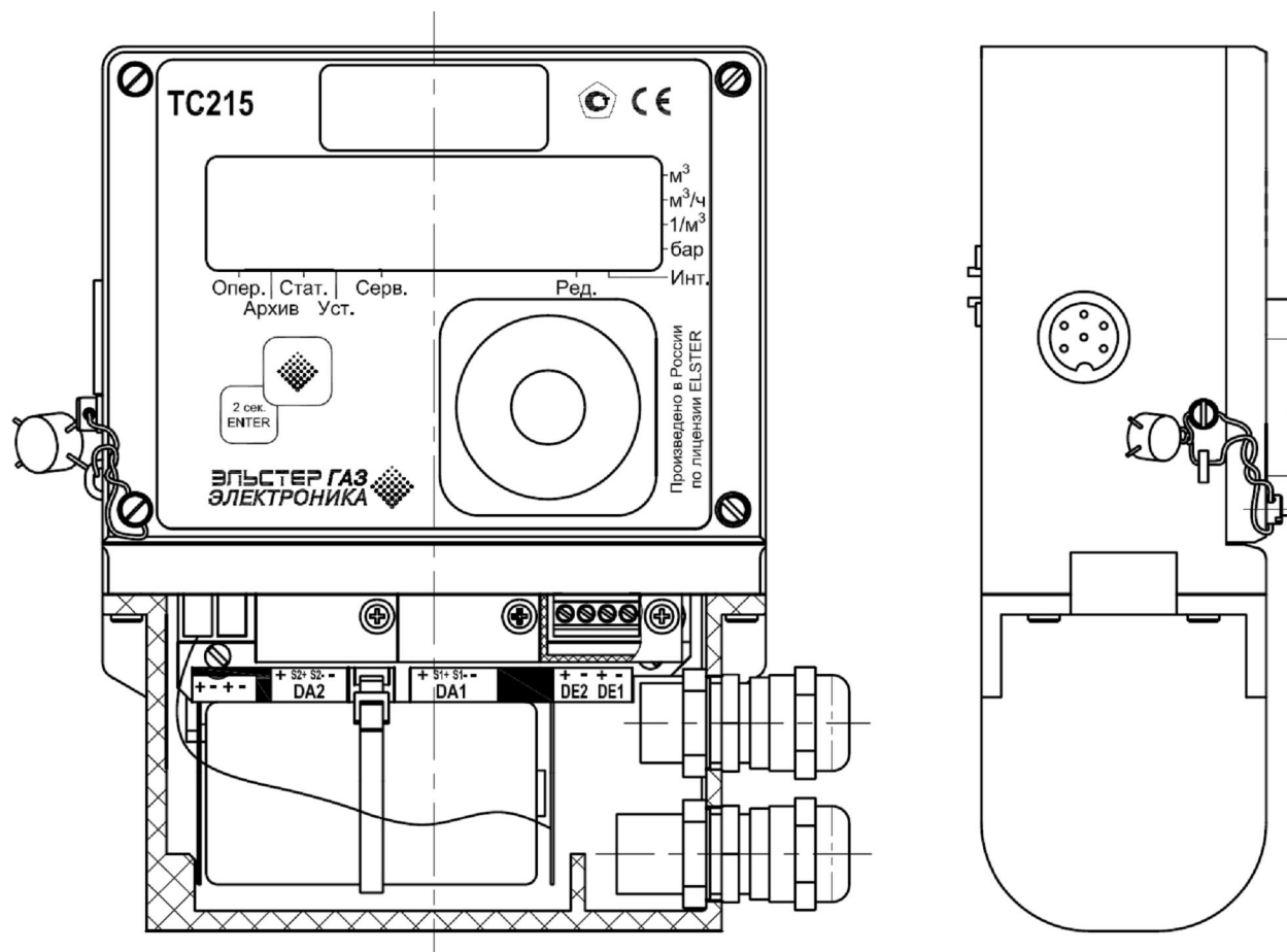
Рис 8. Расположение выводов
